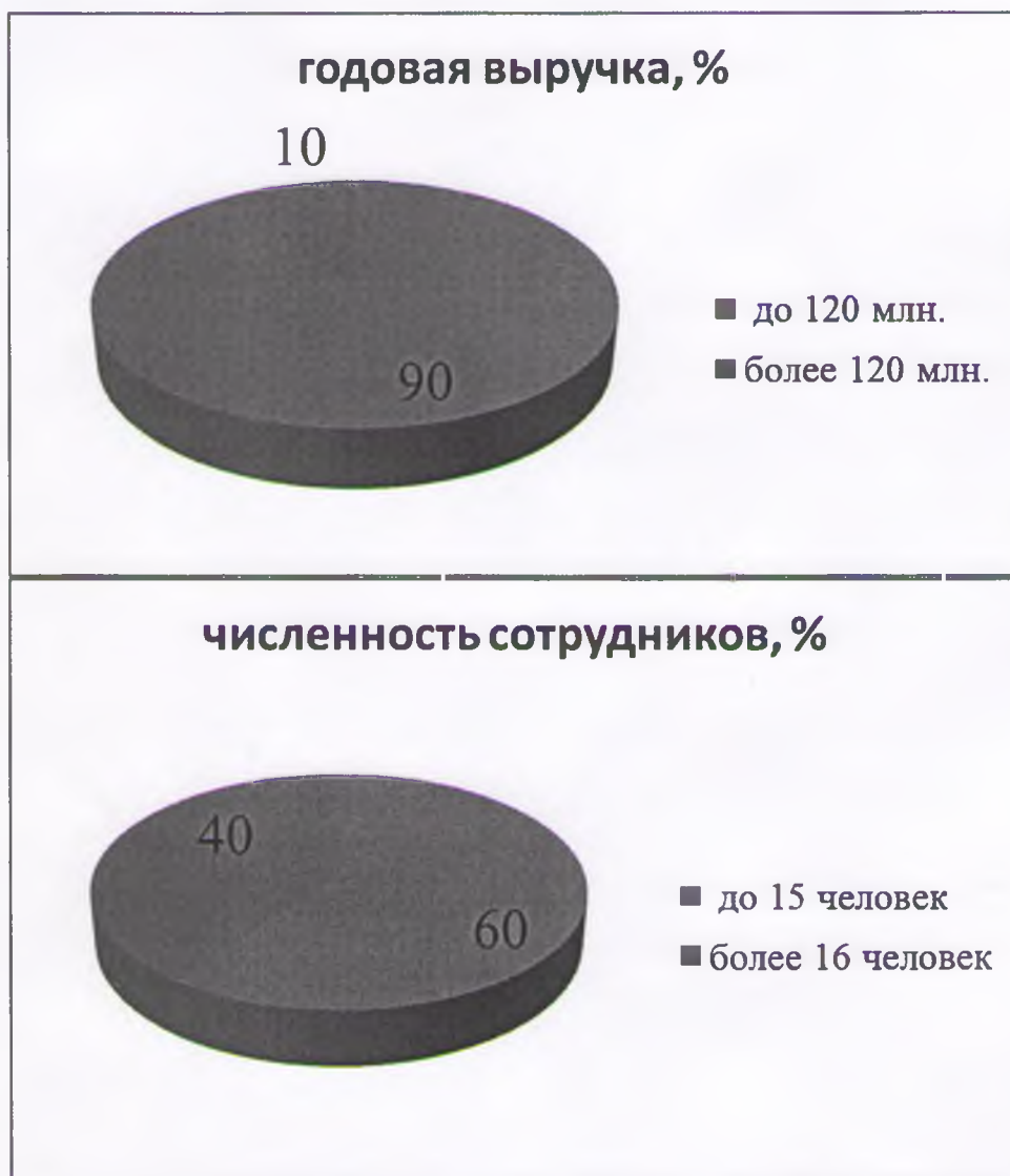
Рисунок 1 – Распределение организаций по годовой выручке и по численности сотрудников организации, % к опрошенным
