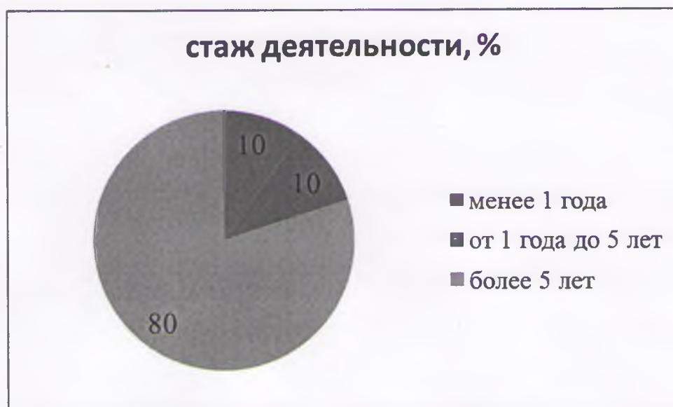
Рисунок 2 – Присутствие организации на рынке, % к опрошенным
